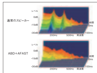
箱内音圧の比較 (実測)
